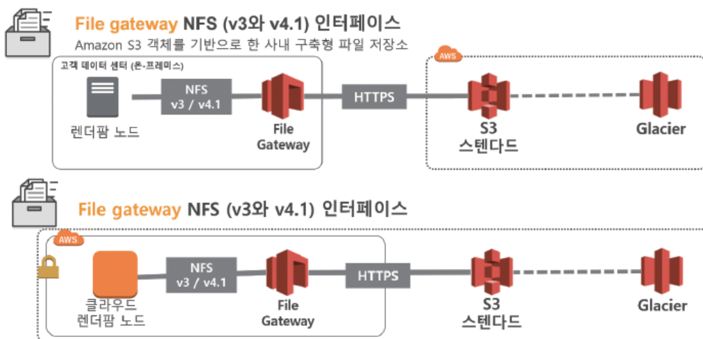
그림 5. AWS Storage Gateway의 File Gateway 기능
