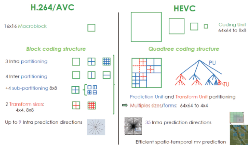
그림 6. H.264와 H.265의 예측 알고리즘 비교
