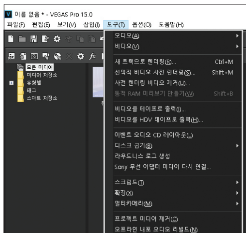
도구 메뉴
