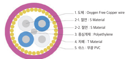
Archest Harmonics 단면 구조
