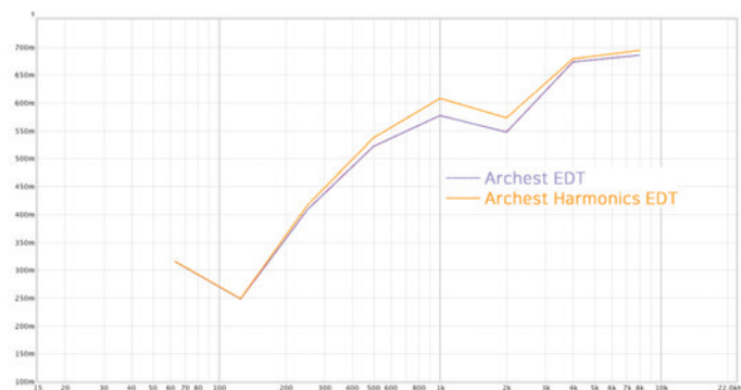
Archest & Archest Harmonics 케이블의 주파수 응답 특성, 흔히 알고 있는 평탄한 모양이 아닌 저음의 명료도를 높이고 중고역대를 풍부하게 재생하도록 리니어한 모양이다.
