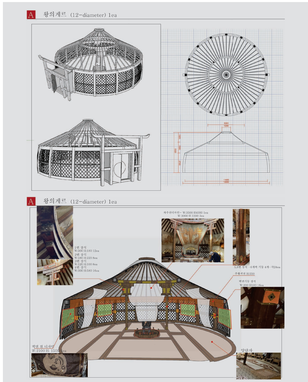
몽골 제작업체에 발주한 작업지시서
